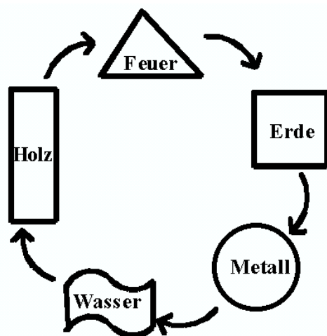
Abbildung 2-7: Erschöpfungszyklus der 5 Elemente
