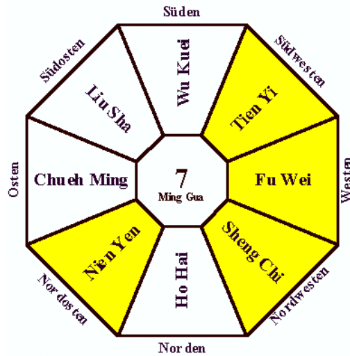
Abbildung 3-5: Lo Shu – Omen für Sonja Eitler
