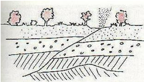
Abbildung 3-2: Geologische Verwerfung
