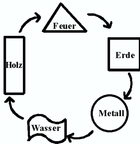
Abbildung 2-5: Entstehungszyklus der 5 Elemente
