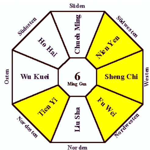
Abbildung 3-7: Ba Zhai für das Wohnhaus
