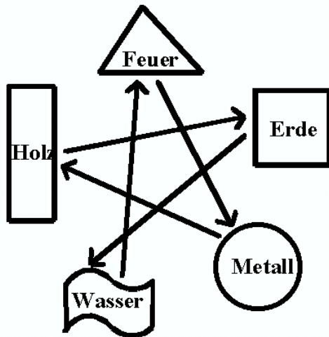
Abbildung 2-6: Kontrollzyklus der 5 Elemente
