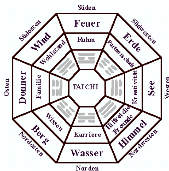
Abbildung 3-14: Ba Gua Bereiche
