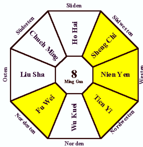
Abbildung 3-6: Lo Shu – Omen für Rupert Kloiber
