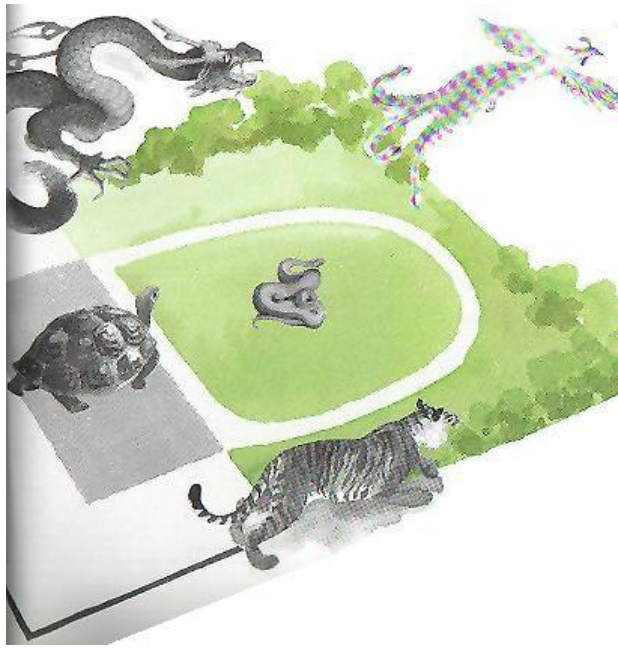
Abbildung 3-3: Die vier Tiere
